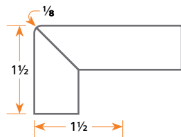
Miter Edge
